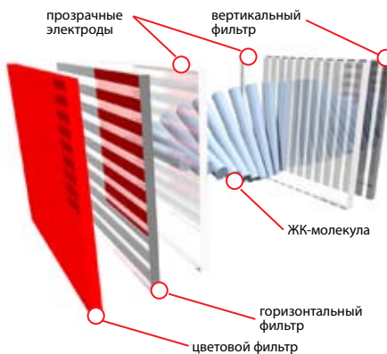
Устройство жидкокристаллической пленки в деталях
